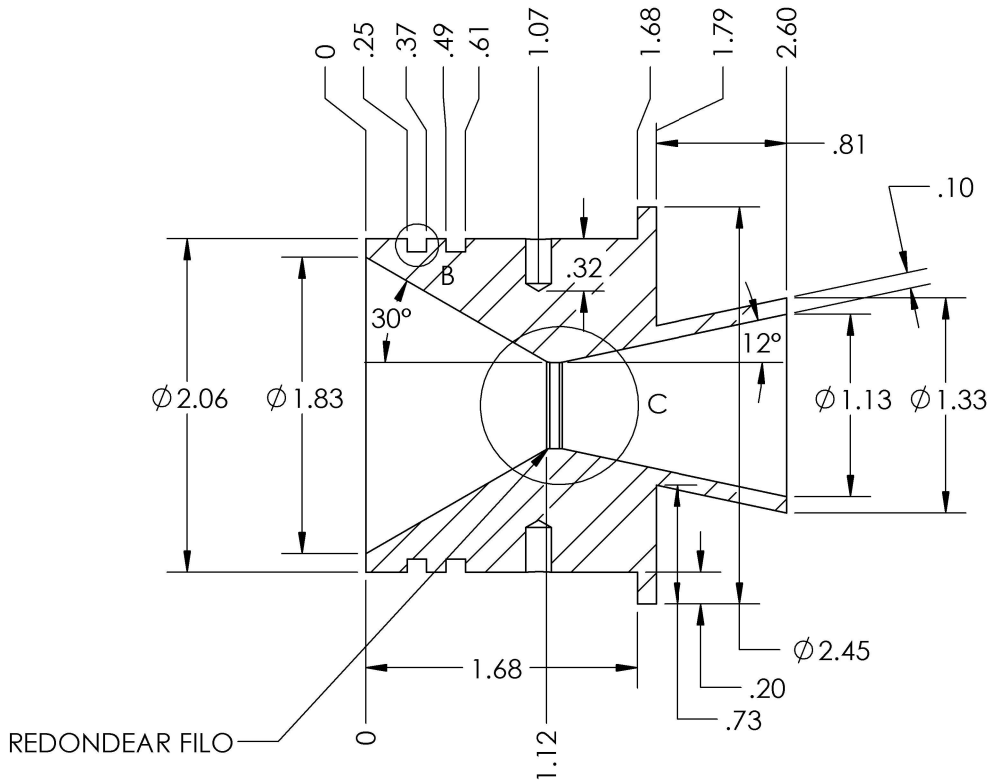
SECCION A-A
