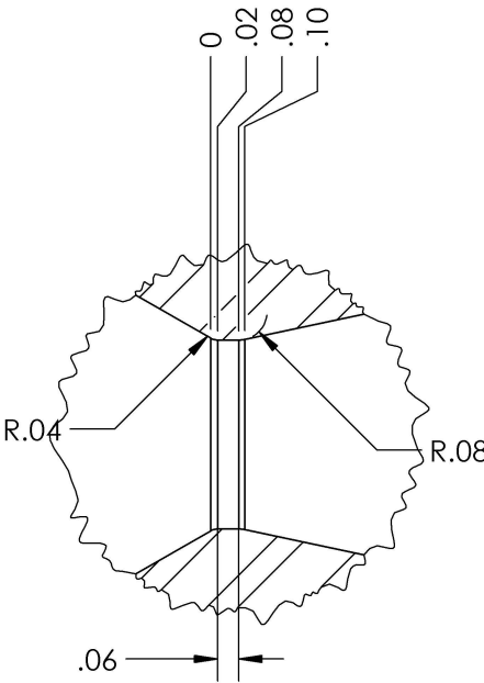
DETALLE C SCALE 2 : 1
