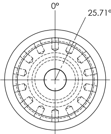
14 BARRENOS M4
